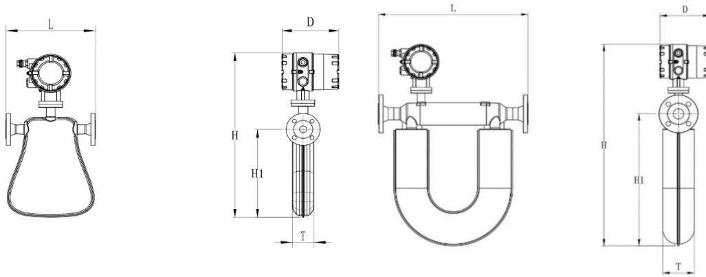
c) 标准一体式，匹配 CFC-100 系列
