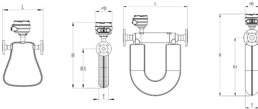
d) 标准分体式，匹配 CFC-030 系列
