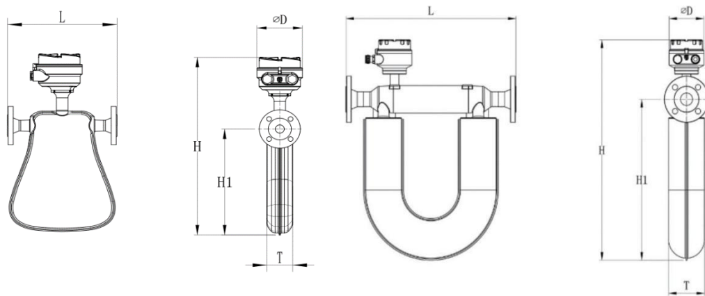
e) 标准分体式，匹配 CFC-100 系列
