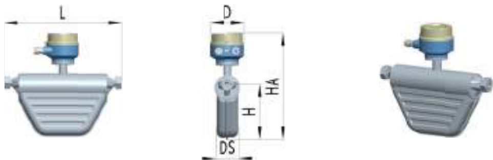
vi、T1/T2/T3版传感器公制尺寸，mm
